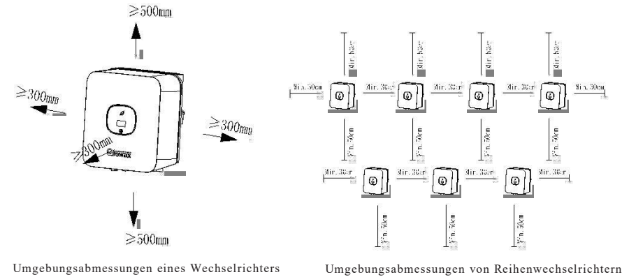
Umgebungsabmessungen eines Wechselrichters
